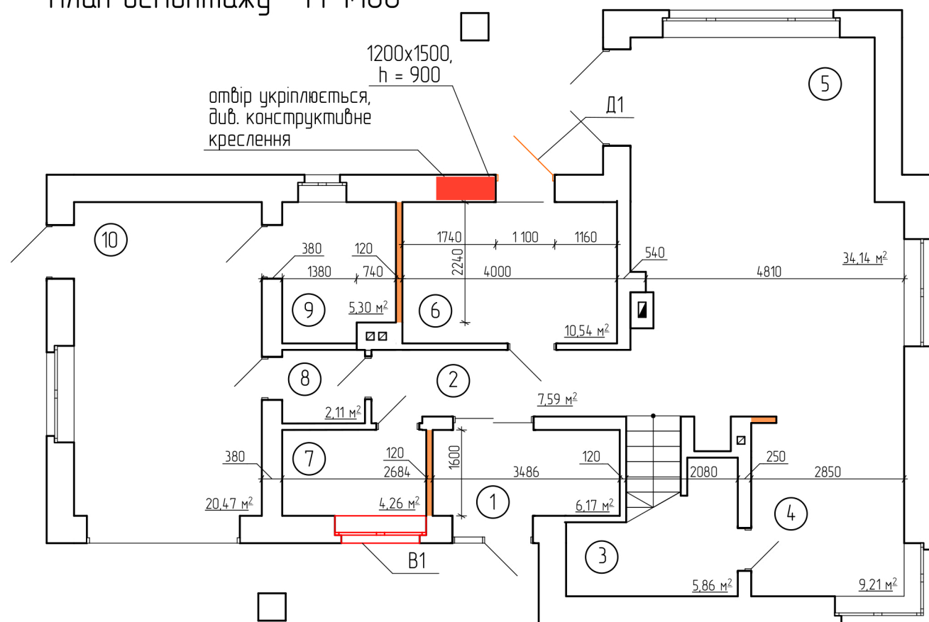
План демонтажу М 1:100
