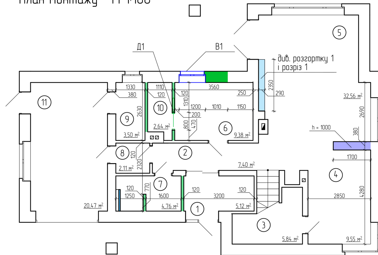
План монтажу М 1:100
