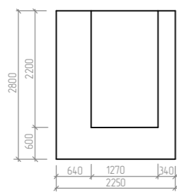
Розгортка А-В
