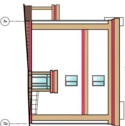
ФАСАД А-В
