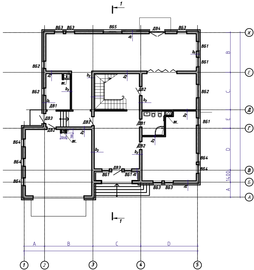
План першого поверху на відм. 0,000
