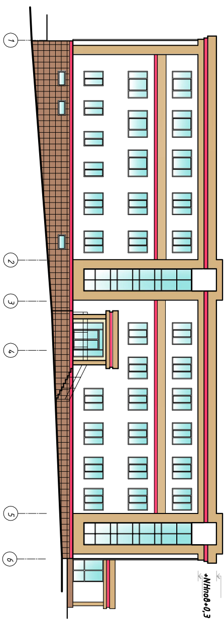
ФАСАД 1-6
