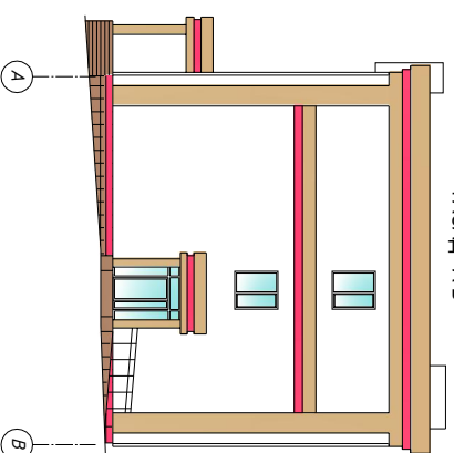
ФАСАД А-В
