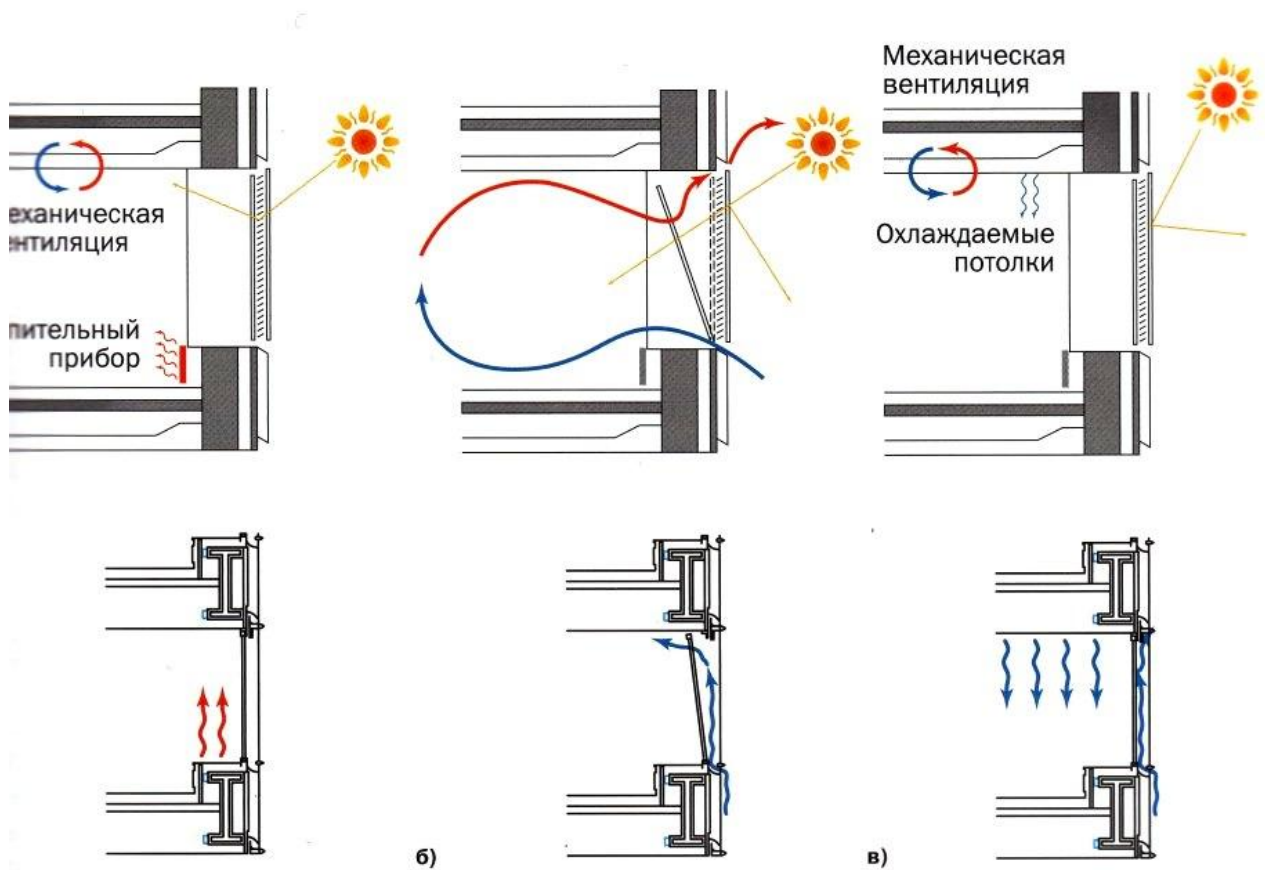
14. Схема климатизации помещения в здании «Commerzbank» в разные периоды года:
