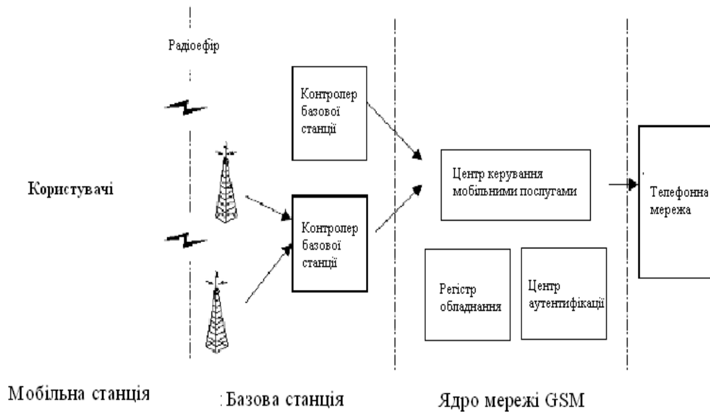
Рисунок 1.9 Структурна схема мережі GSM
