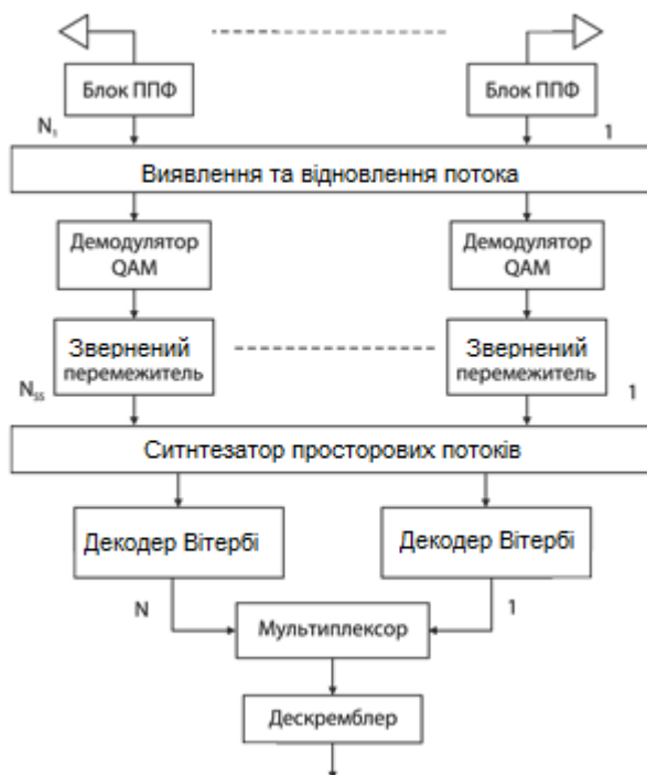
Рисунок 4.5 Загальна структура приймача
