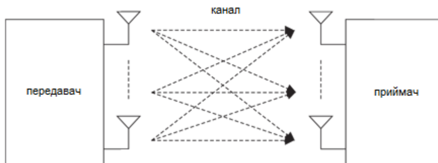
Рисунок 4.3 Принцип реалізації технології MIMO
