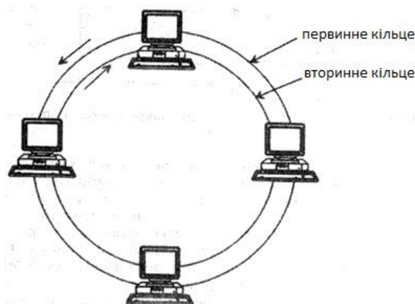
Рисунок 1.4 Стандарт FDDI
