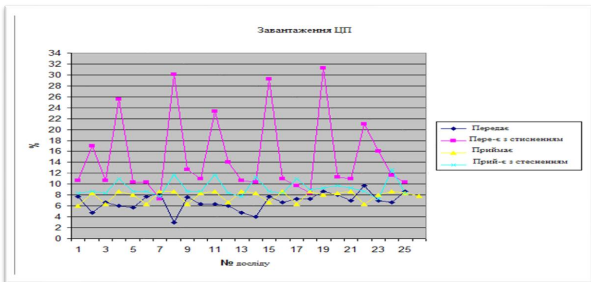
Рисунок 3.4 Графіки завантаження ЦП
