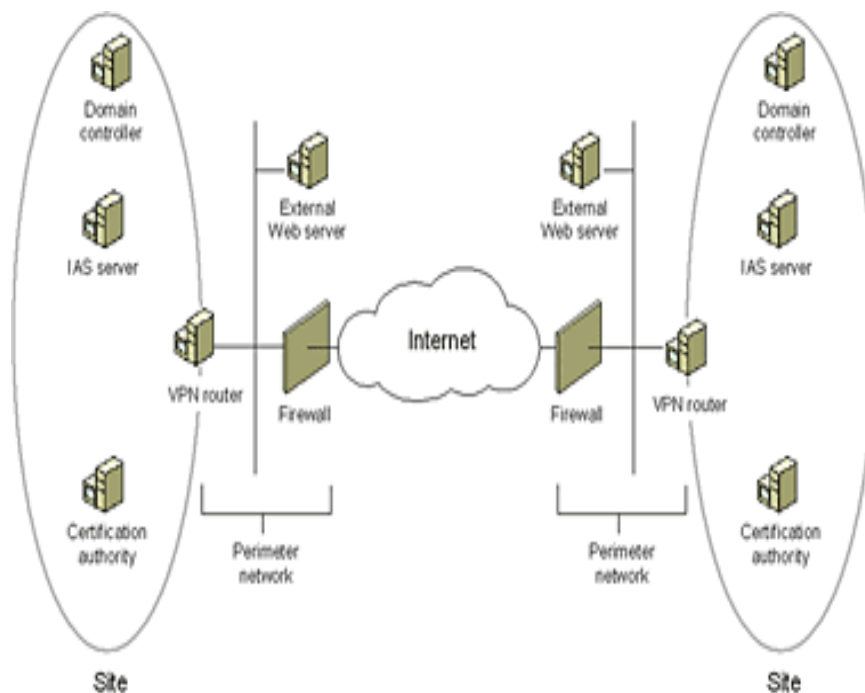
Рисунок 1.5 - Схема побудови VPN на базі брандмауерів
