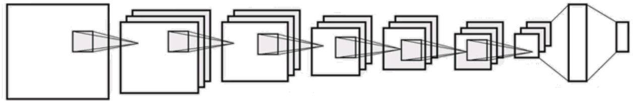
Рис. 1. Структура використаної згорткової нейронної мережі
