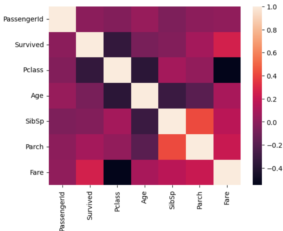
Рисунок 1.19. Теплова карта кореляційного зв'язку
