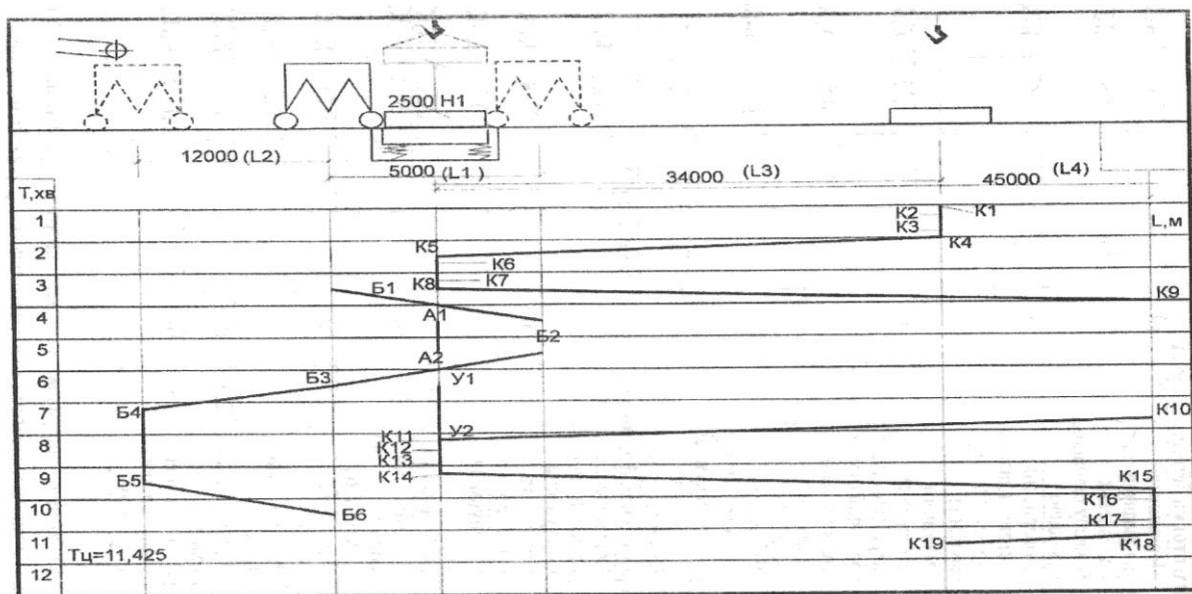
Рис. 5.1. Циклограма роботи обладнання поста формування
