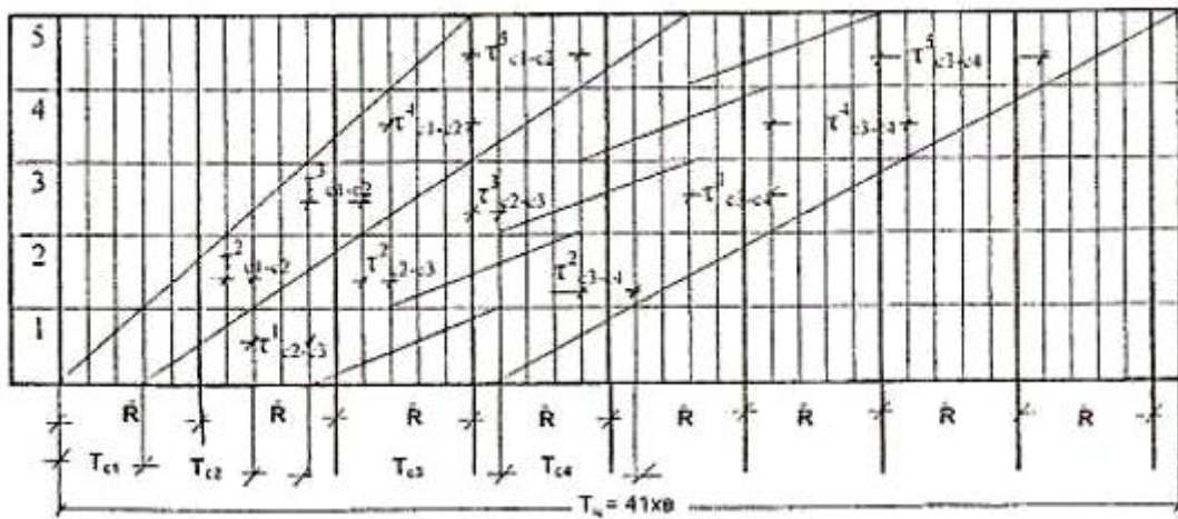
Рис 3.2.Циклограма прямопотокової форми організації часткового процесу: ( \tau^2_{c1-c2} – перерва в обробці другого виробу між першим та другим стадійними прицесами; \tau^3_{c2-c3} – перерва в обробці третього виробу між другим та третім стадійними процесами).
