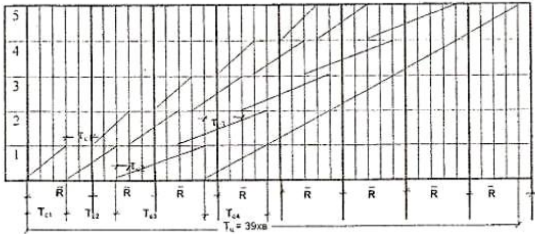
Рис 3.1.Циклограма перервно-потоквої форми організації часткового процесу: ( T_{c1} - T_{c4} – тривалість стадійних процесів; \tau_{c1} , \tau_{c2} , \tau_{c3} – перерви в 1, 2, 3 стадійних процесах).
