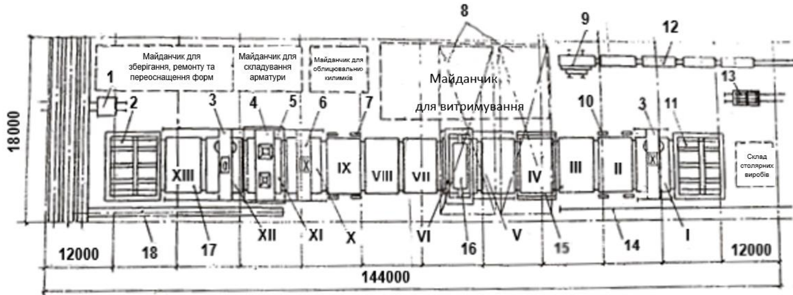
Рис. 1. Конвеєр вертикально-замкнений для виготовлення одношарових зовнішніх стін, які формуються фасадною поверхнею вниз:
