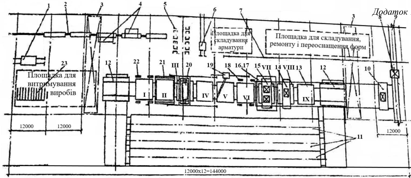
Рис. 8. Конвеєр горизонтально-замкнутий для виготовлення панелей перекриття і внутрішніх стін:
