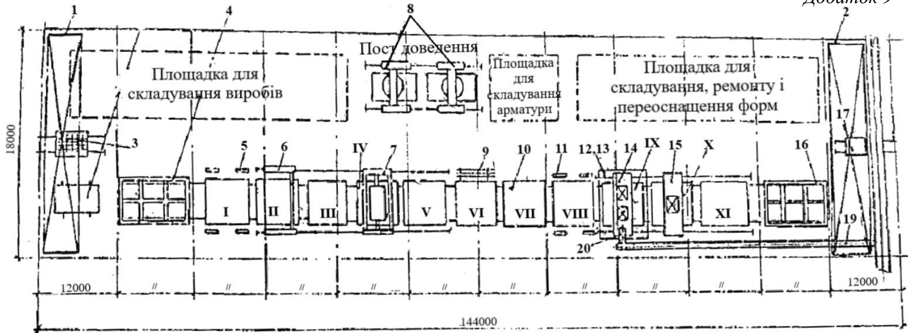
Рис.7. Конвеєр вертикально-замкнений для виготовлення попередньо-напружених панелей перекриття:
