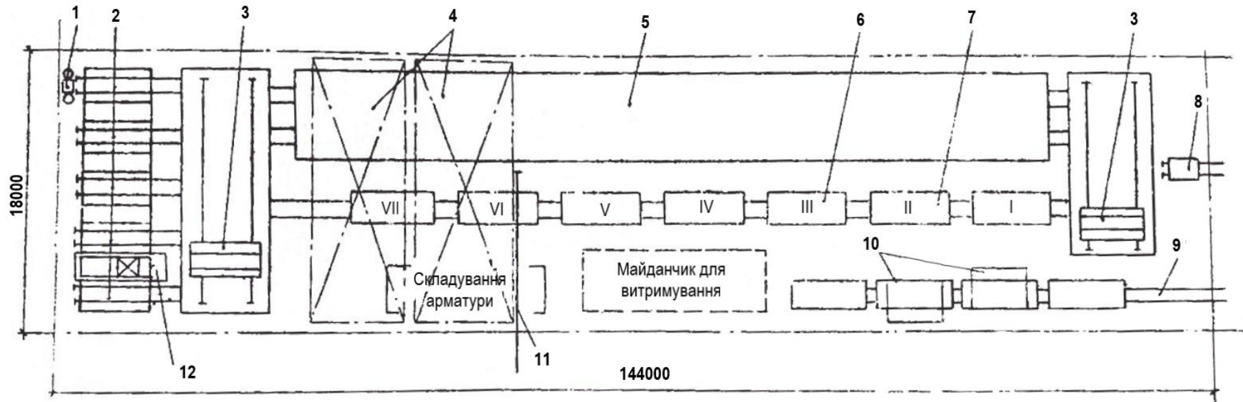
Рис. 10. Технологічна схема виготовлення плит перекриття і панелей внутрішніх стін на касетно-конвеєрній лінії:
