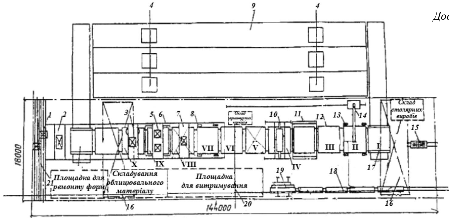
Рис.3. Конвеєр горизонтально-замкнений для виготовлення одношарових панелей зовнішніх стін, які формуються фасадною поверхнею вниз:
