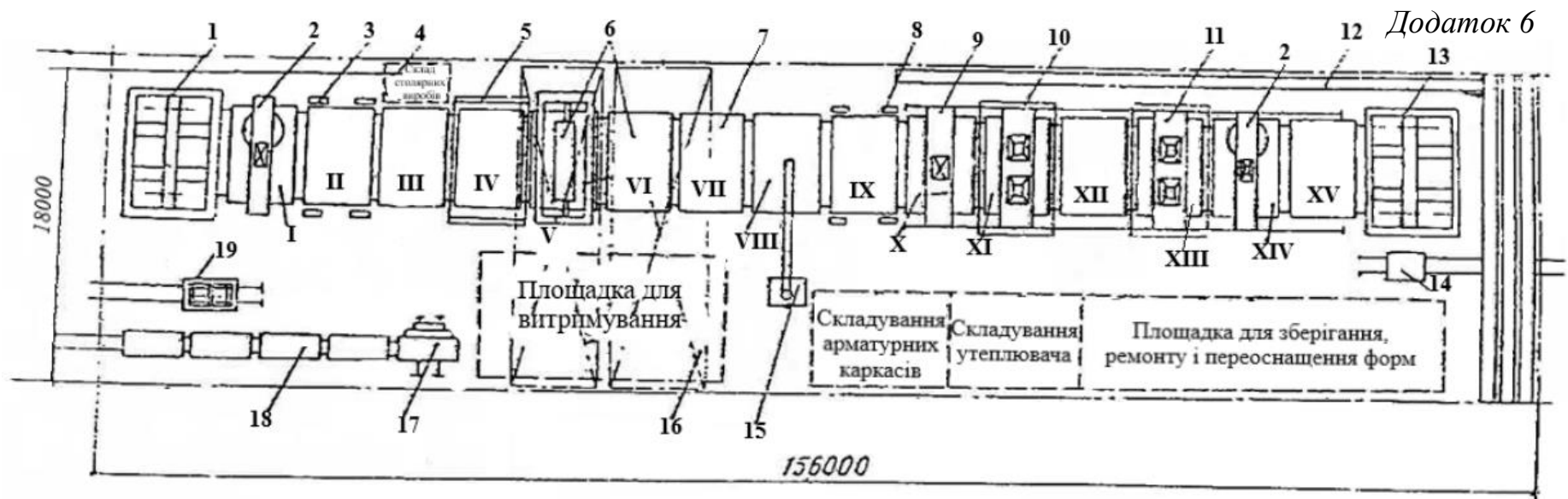
Рис.4. Конвеєр вертикально-замкнутий для виготовлення тришарових панелей зовнішніх стін, які формуються фасадною поверхнею вниз:
