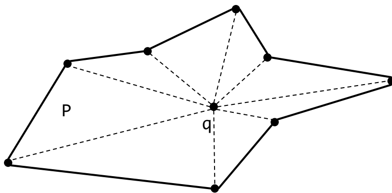
Рис. 11.5. Зірчастий багатокутник
