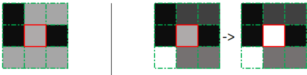
Рис. 15.19. Алгоритм гістерезису
