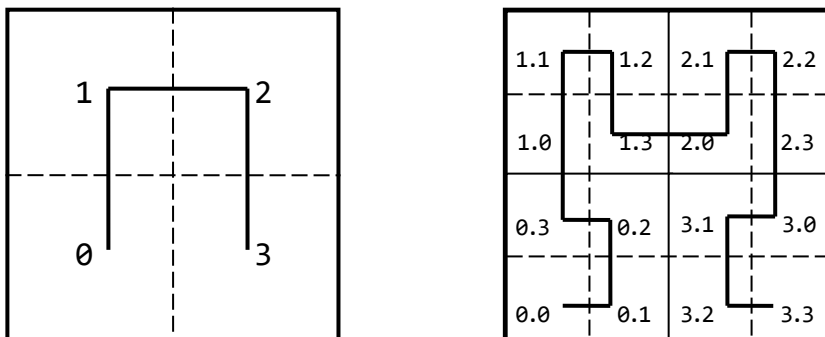
Рис. 12.8. Крива Гільберта
