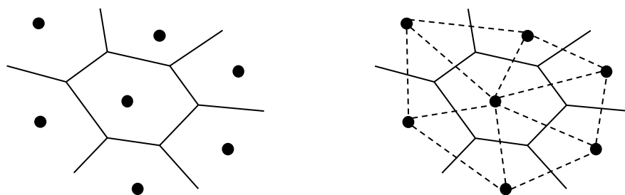
Рис. 7.2. Діаграма Вороного
