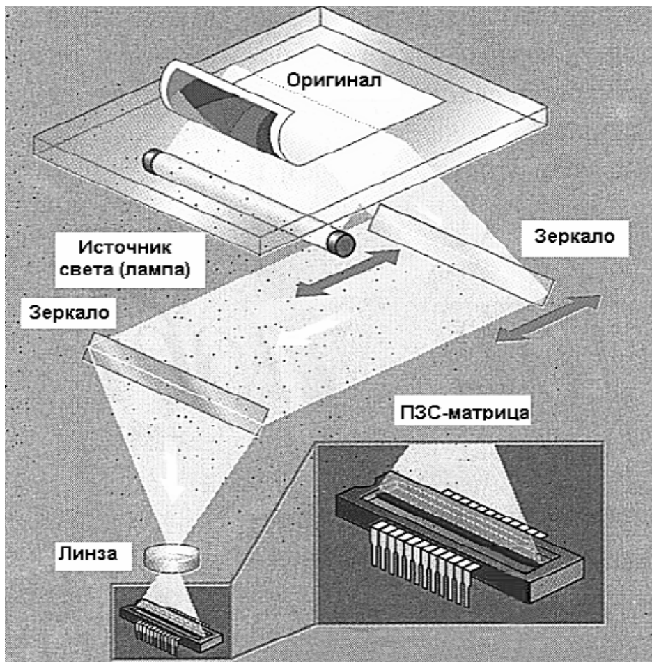
Рисунок 1.6 – Типовий планшетний сканер
