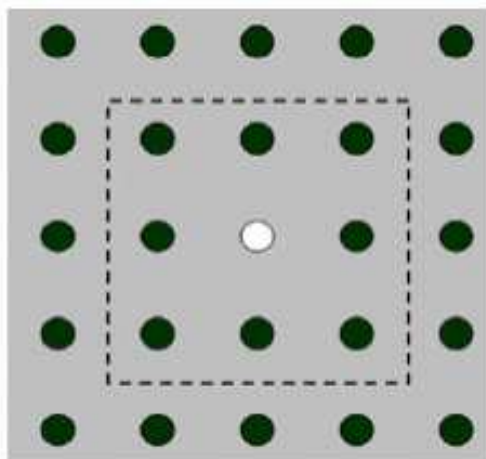
Рисунок 2.8 – Некаузальна модель
