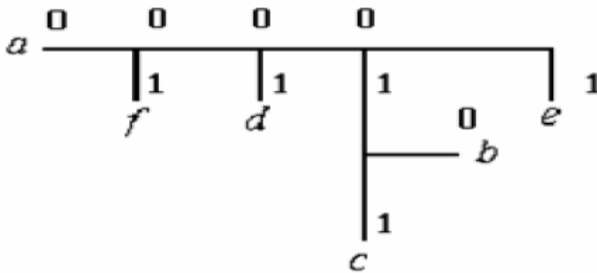
Рисунок 2.4 – Двійкове дерево
