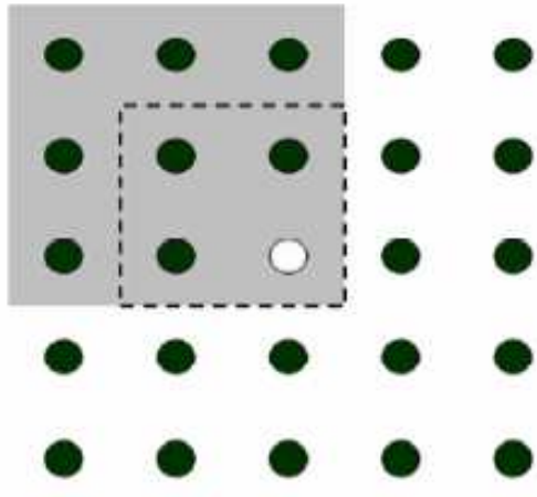
Рисунок 2.5 – Каузальна модель
