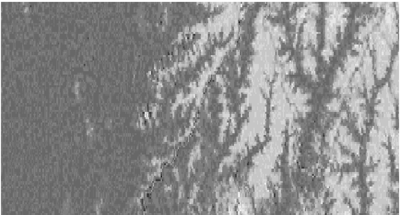
Рисунок 2.14 – Початкове зображення
