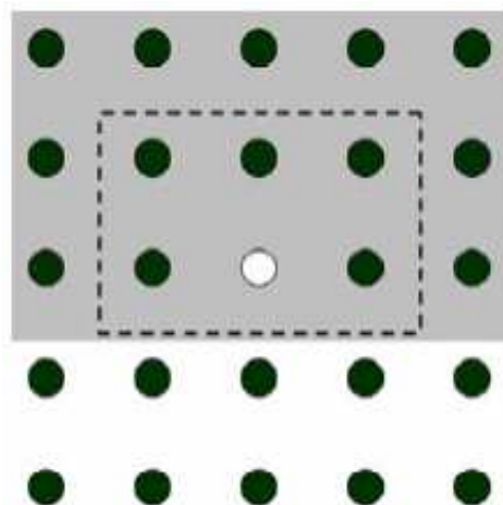
Рисунок 2.7 – Півкаузальна модель
