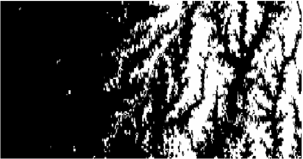
Рисунок 2.15 – Порогова сегментація
