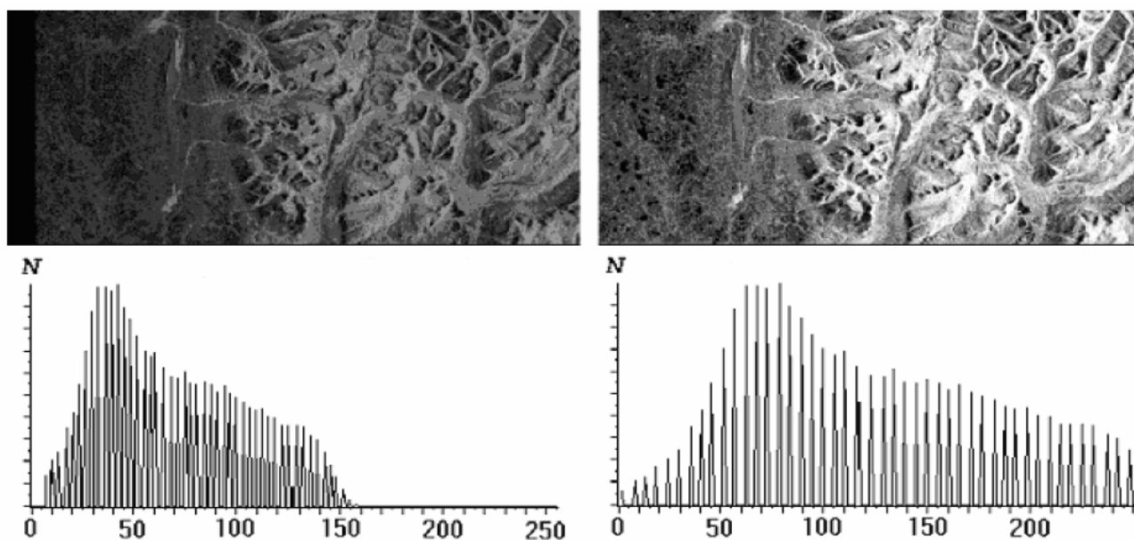
Рисунок 2.12 – Розтяжка гістограми
