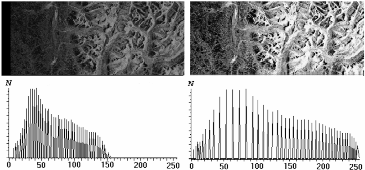
Рисунок 2.13 – Еквалізація гістограми
