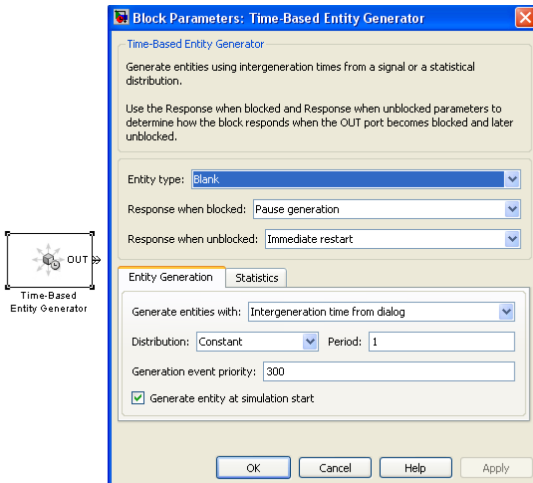
Рис. 18 Блок Time-Based Entity Generator та його діалогове вікно
